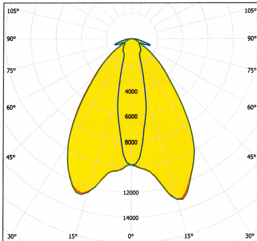
Рисунок 1 – КСС образца светильник светодиодный LED UniLED 80W-LUX-PR*30K в поперечной (C0-C180) (красная кривая), продольной (C90-C270) (синяя кривая) плоскостях и плоскости максимальной силы света (C6-C186) (зеленая кривая)
