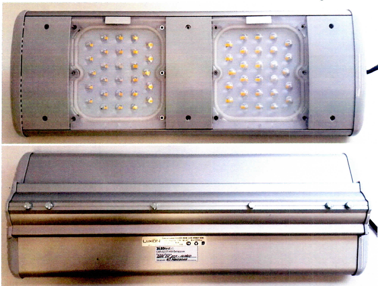
Рисунок 5 – Фотографии образца светильник светодиодный LED UniLED 80W-LUX-PR*30K
