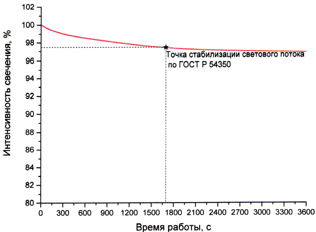
Рисунок 3 – График стабилизации светового потока образца светильник светодиодный LED UniLED 80W-LUX-PR*30K
