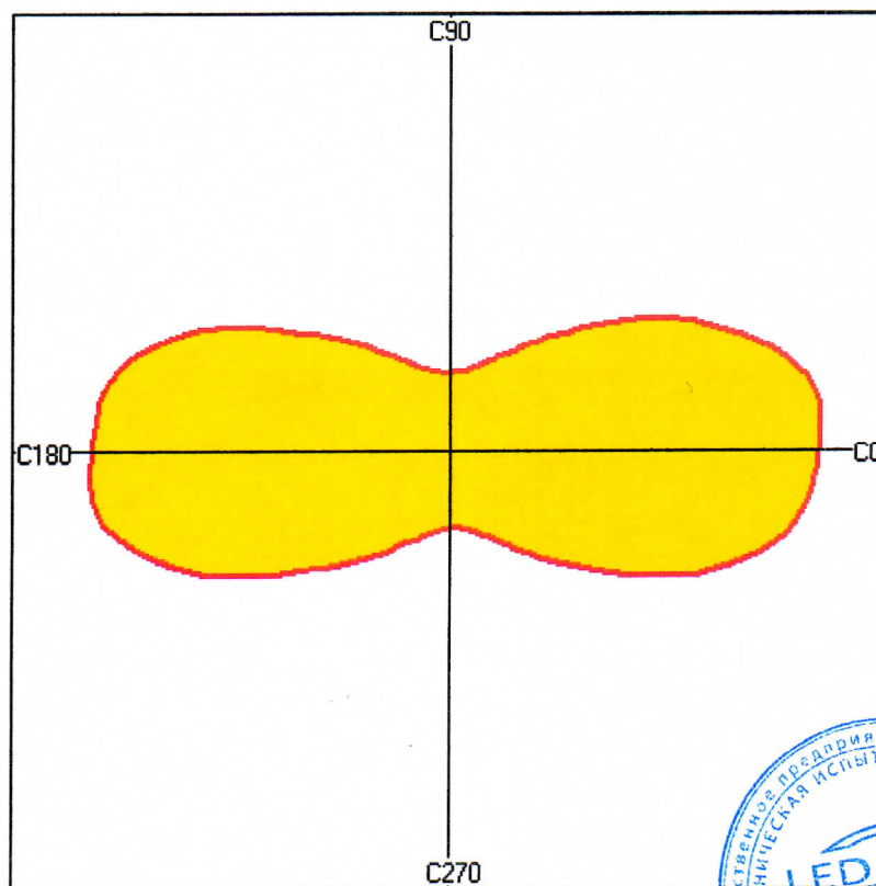
Рисунок 2 – Условная экваториальная КСС образца в направлении максимальной силы света (меридиональный угол 18°)
